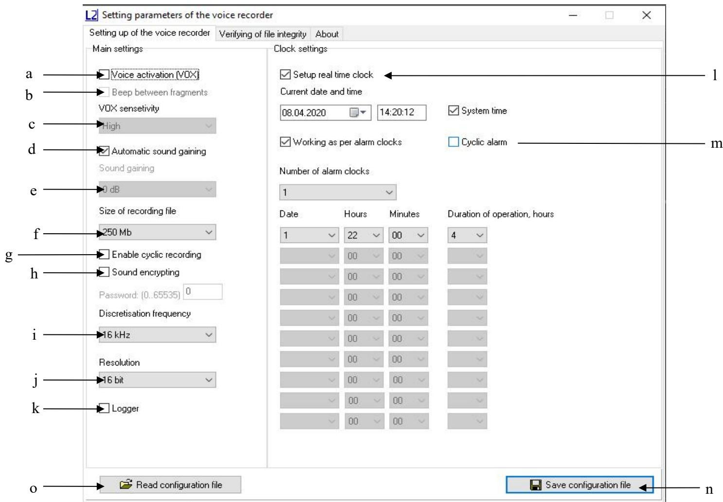
Rys 3. Okno „Setting up the voice recorder”
